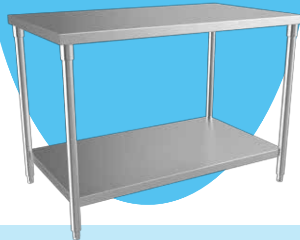
品名：工作台下層板(無背) 尺寸：W1200xD700xH850(mm)
