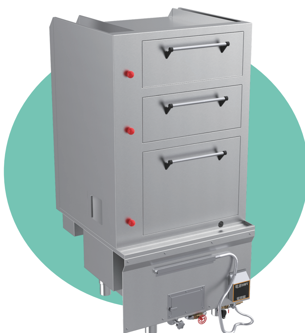
品名：鼓風式港式蒸箱(新型) 尺寸：W950xD850/950xH660/1880(mm) 燃燒室選配升級
