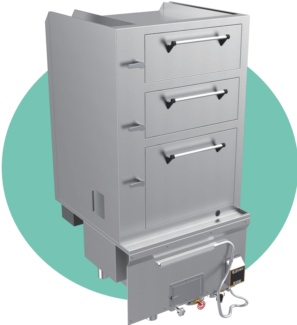
品名：鼓風式港式蒸箱 尺寸：W950xD850/950xH660/1880(mm) 燃燒室選配升級
