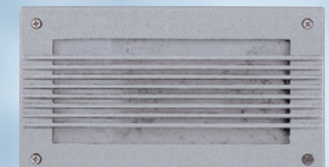
AL26759 3400 W225mm H125mm D80mm E27 小麗晶、LEDx1 另計 鋁合金壓鑄成型、砂灰 噴砂霧面玻璃、附ABS預埋盒 預埋盒：W220mm H120mm D72mm
