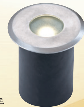
AL26794 4800 W58mm H60mm 附LED 1wx1、暖白、全電壓 鋁合金壓鑄成型、不鏽鋼面蓋、不鏽鋼本色 拋光拉絲處理、噴砂台階玻璃 附鋁合金預埋盒 預埋盒：W43mm H60mm
