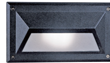
AL26752 1900 W225mm H125mm D100mm E27 小麗晶、LEDx1 另計 鋁合金壓鑄成型、砂黑 噴砂霧面玻璃、ABS預埋盒 另計 預埋盒：W225mm H120mm D77mm
