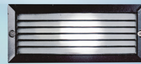
AL26755 1600 W233mm H100mm D83mm E27 小麗晶、LEDx1 另計 鋁合金壓鑄成型、砂黑 噴砂霧面玻璃、ABS預埋盒 另計 預埋盒：W230mm H95mm D76mm
