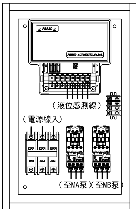
圖示粗線為外接配線處
