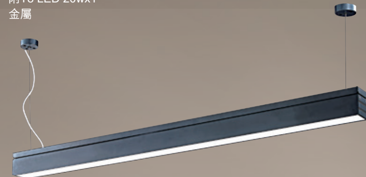
AL24803 10000 L1250mm W70mm H80mm 線長900mm 附T8 LED 20wx1 鋁製品、壓克力
