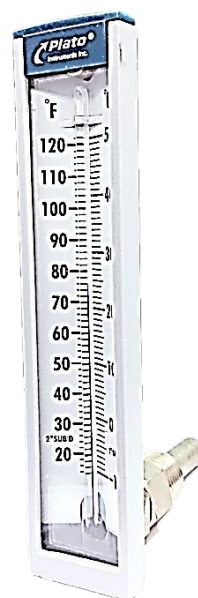
GTP系列 - 塑殼角板型溫度計
