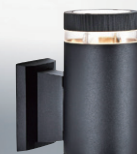
AL26537 3800 W110mm H200mm D155mm E27 LEDx1 另計 鋁合金壓鑄成型、砂黑 透明AC罩
