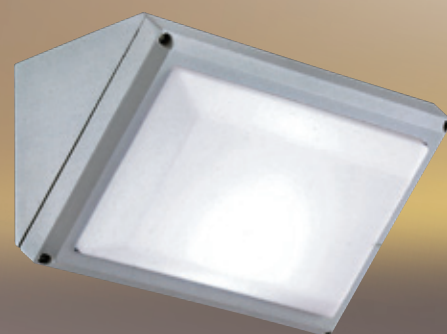
AL26529 6000 W270mm H138mm D140mm E27 LEDx1 另計 鋁合金壓鑄成型、銀灰 乳白AC罩
