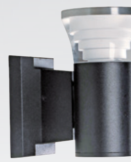
AL2653B 4800 W85mm H150mm D135mm 附LED 3wx1、暖白、全電壓 鋁合金壓鑄成型、砂黑 壓克力
