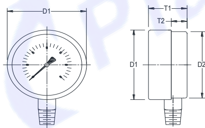
A(直立式)
