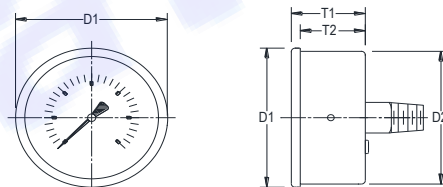
D(埋入式)
