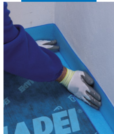
在撕除背面防黏膜後，將Mapesilent Band R繃帶密封，適用所有尺寸的房間
