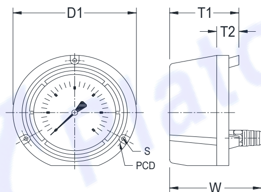
D (埋入式)
