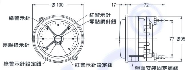
PC (埋入盤面式)
