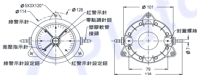
F (牆面壁掛式)
