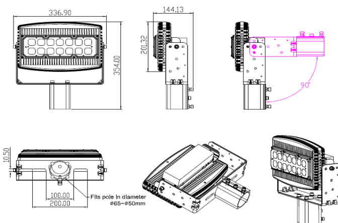
圓桿燈尺寸圖
