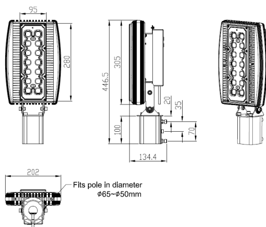
路燈尺寸圖
