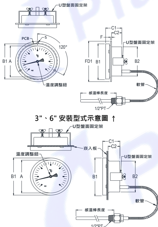
4" 安裝型式示意圖 ↑
