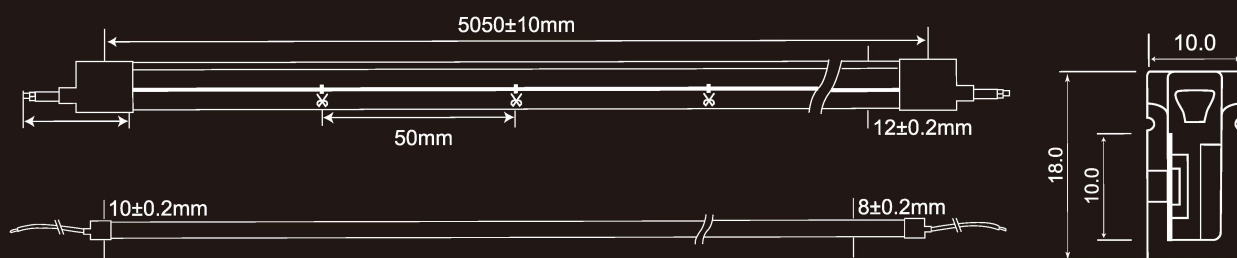
霓虹燈條截面圖
