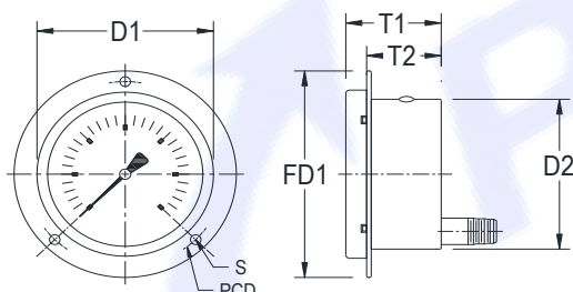
F(埋入式附前緣)
