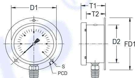
B(直立式附背緣)
