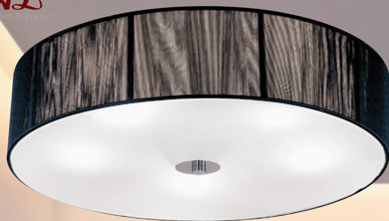
AL24501 10700 W600mm H110mm E27 LEDx6 另計 小夜燈5wx1、附電子開關 鋼材、壓克力、絲罩
