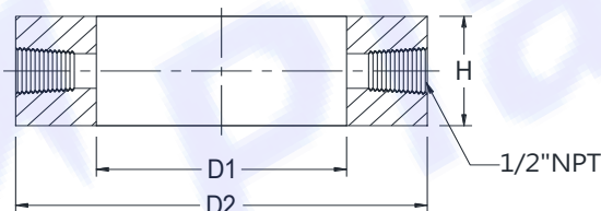
美規 ASME B16.5 規格尺寸表
