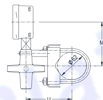
U ( 2"管U環固定式 ↑ )
