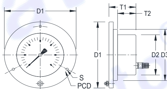
D (埋入式)
