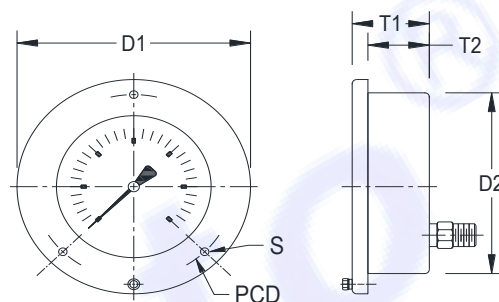
D (埋入式)
