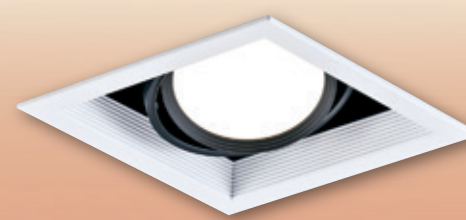
AL25037 3070 L140mm W140mm H140mm 附LED 15wx1 附美國 CREE 晶片、全電壓 3000K、4000K、5700K、防眩光
