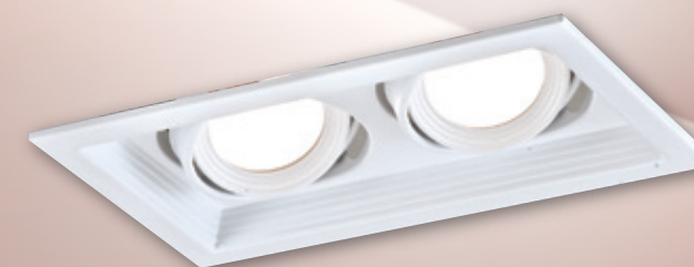
AL25034 4340 L225mm W130mm H120mm 附LED 12wx2 附美國 CREE 晶片、全電壓 3000K、4000K、5700K、防眩光
