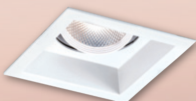
AL2506C 3600 L135mm W135mm H120mm 附 CREE CXA COB 18w模組x1 3000K、4000K、5700K 鋁材、粉體烤漆
