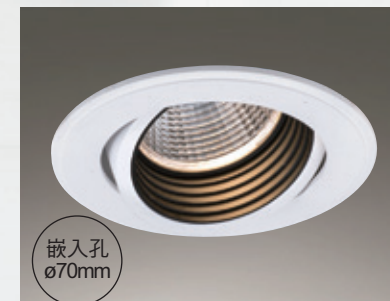
AL25075 2500 W85mm H70mm 附 CREE CXA COB 10w 3000K、4000K、5700K 鋁材、粉體烤漆
