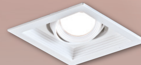
AL25033 2340 L130mm W130mm H120mm 附LED 12wx1 附美國 CREE 晶片、全電壓 3000K、4000K、5700K、防眩光
