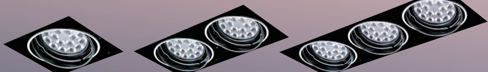
AL2502A 4670 L161mm W161mm H90mm 附高亮度原裝進口 OSRAM LED 22wx1 AC100V-240V (台灣電子) 3000K、流明2700Lm 鋼材 (台灣製造) 無邊框請準確開孔
