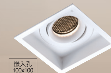
AL2507D 3900 L111mm W111mm H125mm 附 CREE CXA 18w模組 3000K、4000K、5700K 鋁材、粉體烤漆
