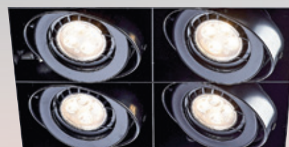
AL25069 7800 L206mm W206mm H85mm 附LED 4珠 6wx4 OSRAM 3030 / 3000K、4000K、5700K 鋼鐵鋁材、粉體烤漆、無邊框請準確開孔
