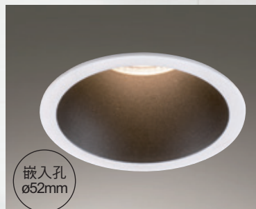
AL25076 2400 W60mm H85mm 附 CREE CXA COB 10w 3000K、4000K、5700K 鋁材、粉體烤漆
