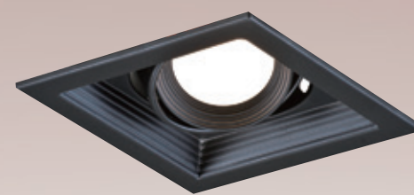
AL25035 2340 L130mm W130mm H120mm 附LED 12wx1 附美國 CREE 晶片、全電壓 3000K、4000K、5700K、防眩光
