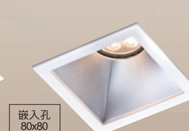
AL2507F 1800 L84mm W84mm H110mm 附 OSRAM 3030x6珠 8w 3000K、4000K、5700K 鋁材、工程塑膠、粉體烤漆
