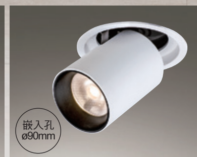
AL25073 3900 W97mm H97mm 附 CREE CXA COB 15w 3000K、4000K 鋁材、粉體烤漆、伸縮投嵌
