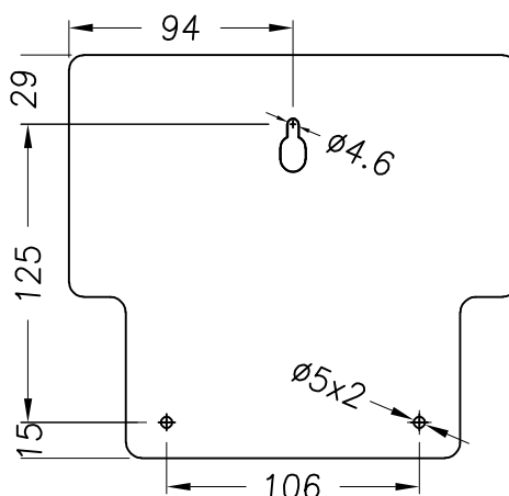
背視圖
