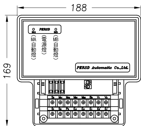
正視圖
