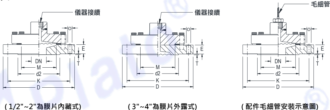
德規 DIN EN 1092-1 規格尺寸表
