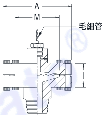
( 配件毛細管安裝示意圖 )
