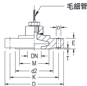
(配件毛細管安裝示意圖)
