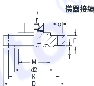
(2"~4"為膜片外露式)
