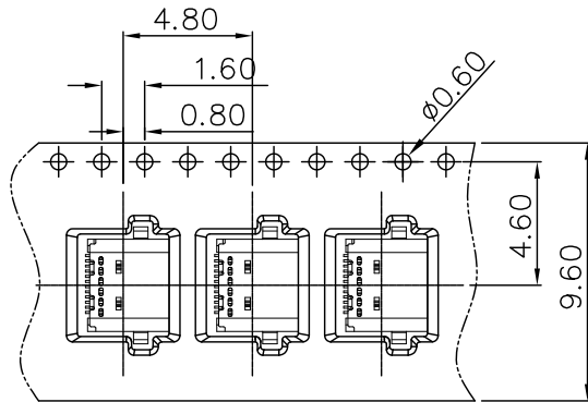
① 产品入载带示意图
