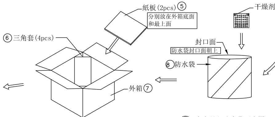
⑤ 产品入外箱示意图
