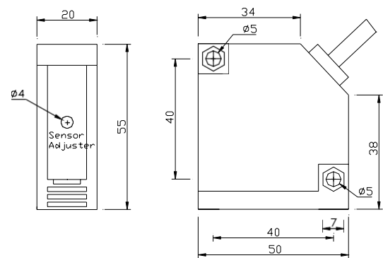
導線引出型
