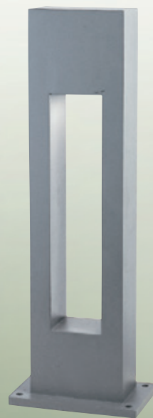
AL26603 18400 W190mm H800mm 底座265mm E27 LEDx1 另計 鋁合金壓鑄成型、砂灰 透明平板玻璃
