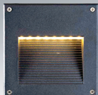
AL26723 4200 L160mm W160mm H94mm 附LED 3wx1、暖白、全電壓 鋁合金壓鑄成型、砂黑 噴砂霧面玻璃、附ABS預埋盒 預埋盒：L160mm W160mm H94mm
