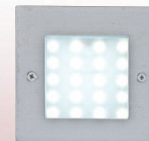
AL26734 3600 W105mm H105mm D60mm 附LED 2wx1、暖白、全電壓 鋁合金壓鑄成型、不鏽鋼面蓋 不鏽鋼本色、拋光拉絲處理 噴砂玻璃、附ABS預埋盒 預埋盒： W95mm H95mm D52mm
