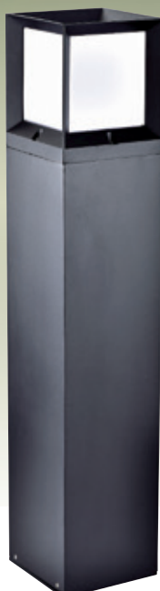
AL2660A 16400 L160mm W160mm H800mm E27 LEDx1 另計 鋁合金組裝成型、砂黑 奶白PC罩
