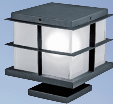
AL26664 18400 L250mm W250mm H270mm E27 LEDx1 另計 不鏽鋼焊接組裝成型、平光黑 噴砂玻璃
