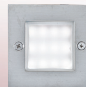
AL26733 2400 W70mm H70mm D55mm 附LED 1wx1、暖白、全電壓 鋁合金壓鑄成型、不鏽鋼面蓋 不鏽鋼本色、拋光拉絲處理 噴砂玻璃、附ABS預埋盒 預埋盒： W62mm H62mm D50mm
