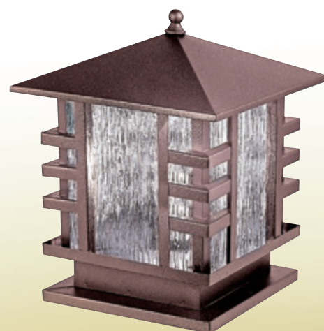
AL26582 8600 L300mm W300mm H380mm E27 LEDx1 另計 金屬鐵材焊接成型、黑咖啡 條紋玻璃
