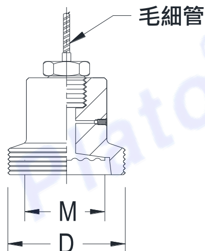
(配件毛細管安裝示意圖)
