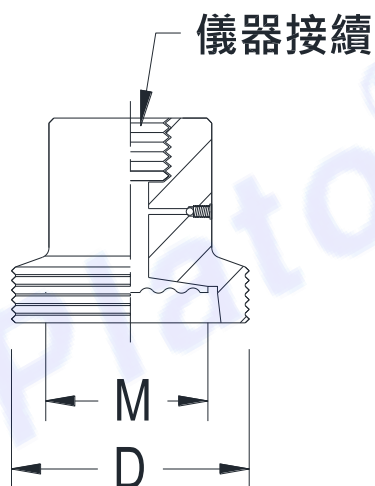
(尺寸示意圖)
