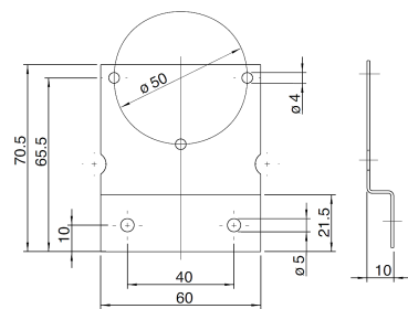
Befestigungswinkel 6402
