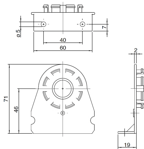
Befestigungswinkel 6482
