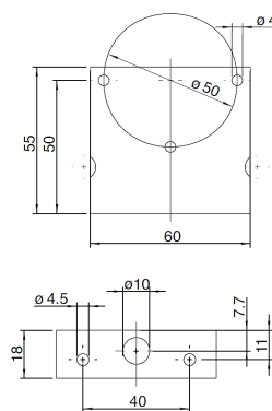
Befestigungswinkel 6401
