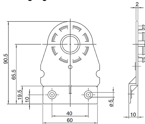
Befestigungswinkel 6482
