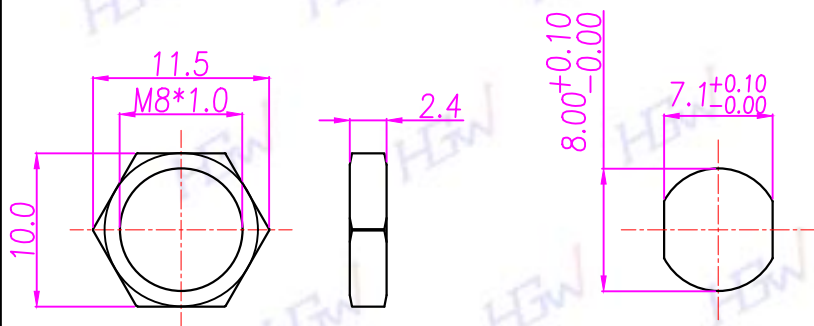
NUT
