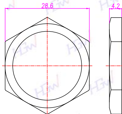
Hex Nut
