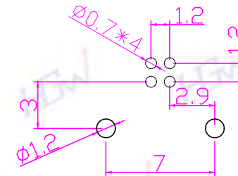
P.C.B LAYOUT
