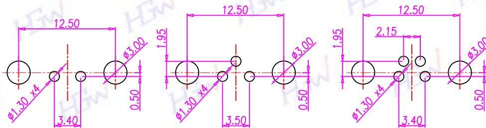
P.C.B. LAYOUT
