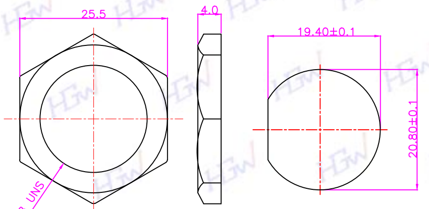
Hex Nut
