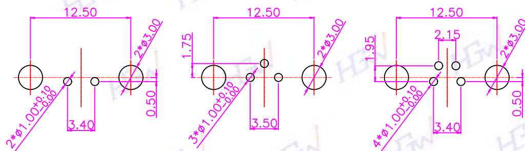
RECOMMEND P.C.B LAYOUT
