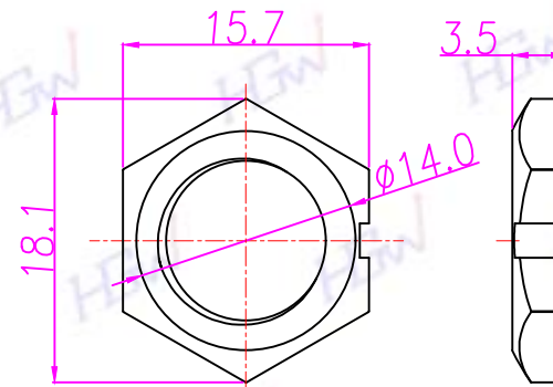
HEX NUT
