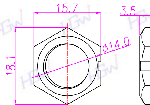
HEX NUT
