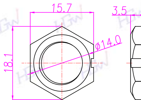
HEX NUT
