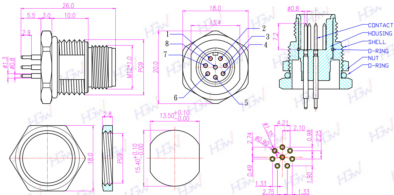
NUT(SEE TABLE A)
