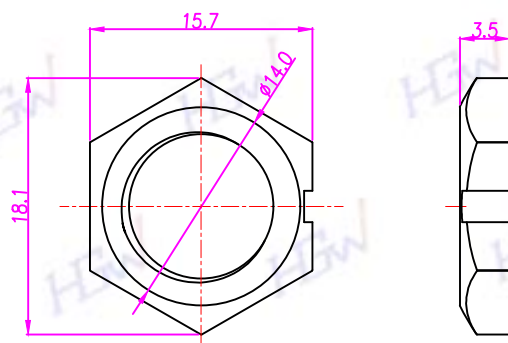
HEX NUT
