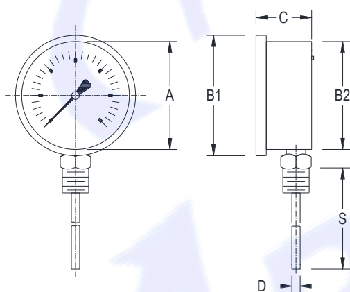
正面示意圖
