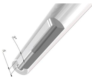
EZSR=3度斜角細型 EZSR=3° SlimRegular
