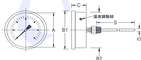
正面示意圖
