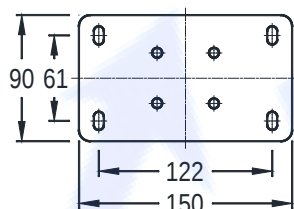
A ( 壁掛固定式 ↑ )
