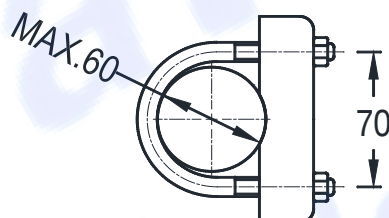
U ( 2"管U環固定式 ↑ )
