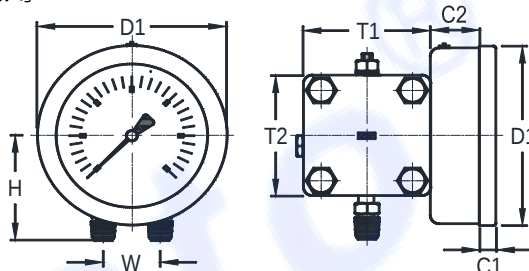
( 6" 不銹鋼差壓錶 ↑ )
