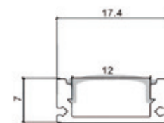
AL25275 2000 W17.4mm H7mm 附LED 2835條燈 變壓器依瓦數搭配另計 以1米計價 鋁製品、壓克力
