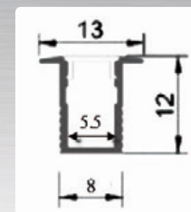
嵌入孔 ø8mm AL25272 2000 W13mm H12mm 附LED 2835條燈 變壓器依瓦數搭配另計 以1米計價 鋁製品、壓克力
