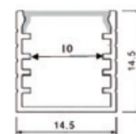
AL25274 2000 W14.5mm H14.5mm 附LED 2835條燈 變壓器依瓦數搭配另計 以1米計價 鋁製品、壓克力
