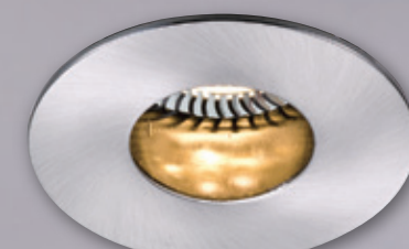
嵌入孔 ø70mm AL25252 1400 W85mm H85mm 附MR16 LED 8wx1 OSRAM 燈珠 發光效率110LM/W 鋁製品
