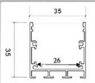
AL25262 2340 W35mm H35mm 附LED 2835條燈 變壓器依瓦數搭配另計 以1米計價 鋁製品、壓克力
