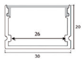
AL25261 2000 W30mm H20mm 附LED 2835條燈 變壓器依瓦數搭配另計 以1米計價 鋁製品、壓克力
