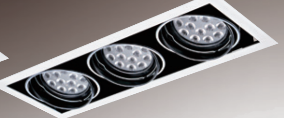
AL25159 12000 L482mm W182mm H90mm 附高亮度原裝進口 OSRAM LED 18wx3 AC100V-240V (台灣電子) 3000K / 流明6750Lm 鋼材、台灣製造
