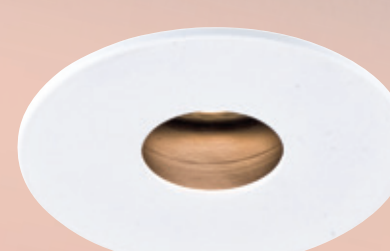
嵌入孔 ø85mm AL25258 2000 W96mm H40mm 附MR16 LED 8wx1 OSRAM 燈珠 發光效率110LM/W OSRAM 8w可雙層分離拆裝 鋁製品
