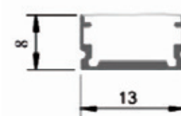
AL25273 2000 W13mm H8mm 附LED 2835條燈 變壓器依瓦數搭配另計 以1米計價 鋁製品、壓克力
