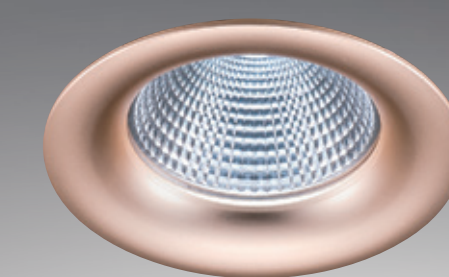
嵌入孔 ø90mm AL25217 1740 W105mm H50mm 附LED 7wx1 附美國普瑞晶片、全電壓 3000K / 4000K / 6000K
