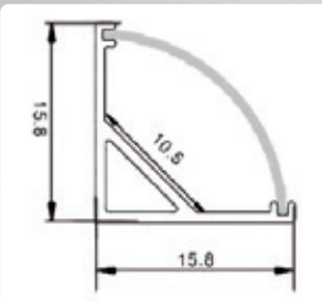
AL25271 2000 W15.8mm H15.8mm 附LED 2835條燈 變壓器依瓦數搭配另計 以1米計價 鋁製品、壓克力
