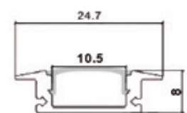
嵌入孔 ø18mm AL25264 2000 W24.7mm H8mm 附LED 2835條燈 變壓器依瓦數搭配另計 以1米計價 鋁製品、壓克力
