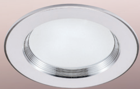
嵌入孔 ø85mm AL25207 670 W98mm H45mm 附LED 5wx1、全電壓 白光、黃光、自然光可3段切換
