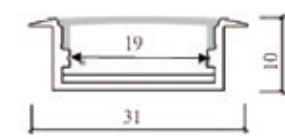
嵌入孔 ø24mm AL25265 2000 W31mm H10mm 附LED 2835條燈 變壓器依瓦數搭配另計 以1米計價 鋁製品、壓克力
